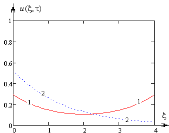
1 – после реверса воздушного потока ( \tau_1 = 0.4 ); 2 – в отсутствии реверса
