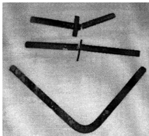
Рис. 7. Испытанные образцы из стали марки СтЗсп
