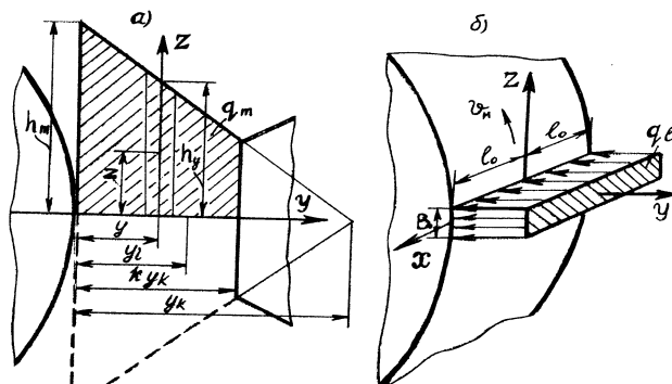
Рис. 2. Расчетные схемы температурных полей от объемного источника тепловыделения (а) и полосового быстро движущегося источника (б)
