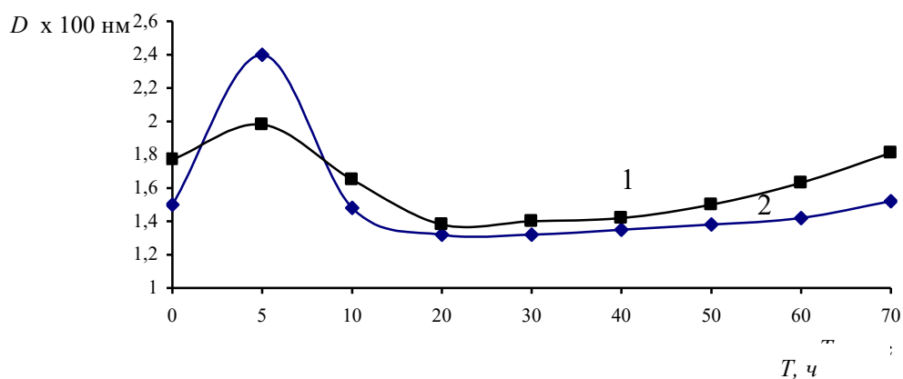
Рис. 3. Изменение среднего диаметра D дисперсных частиц битумов БН/10 (1) и БНД 90/130 (2) в зависимости от продолжительности T их термообработки.
