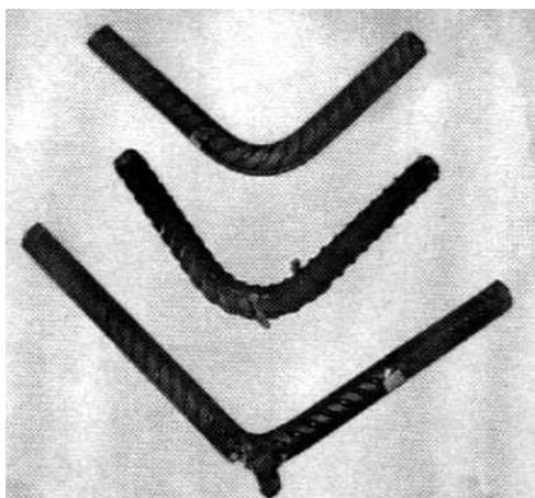
Рис. 6. Испытанные образцы из стали марки 35ГС
