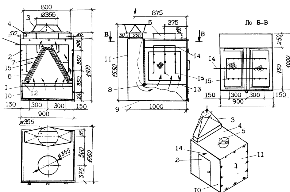
Рис. 1. Конструкция тканевого фильтра:
